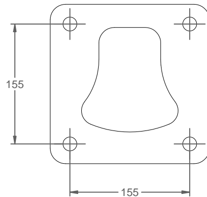
vista en planta 1:5
