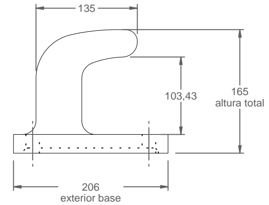
vista lateral 1:5
